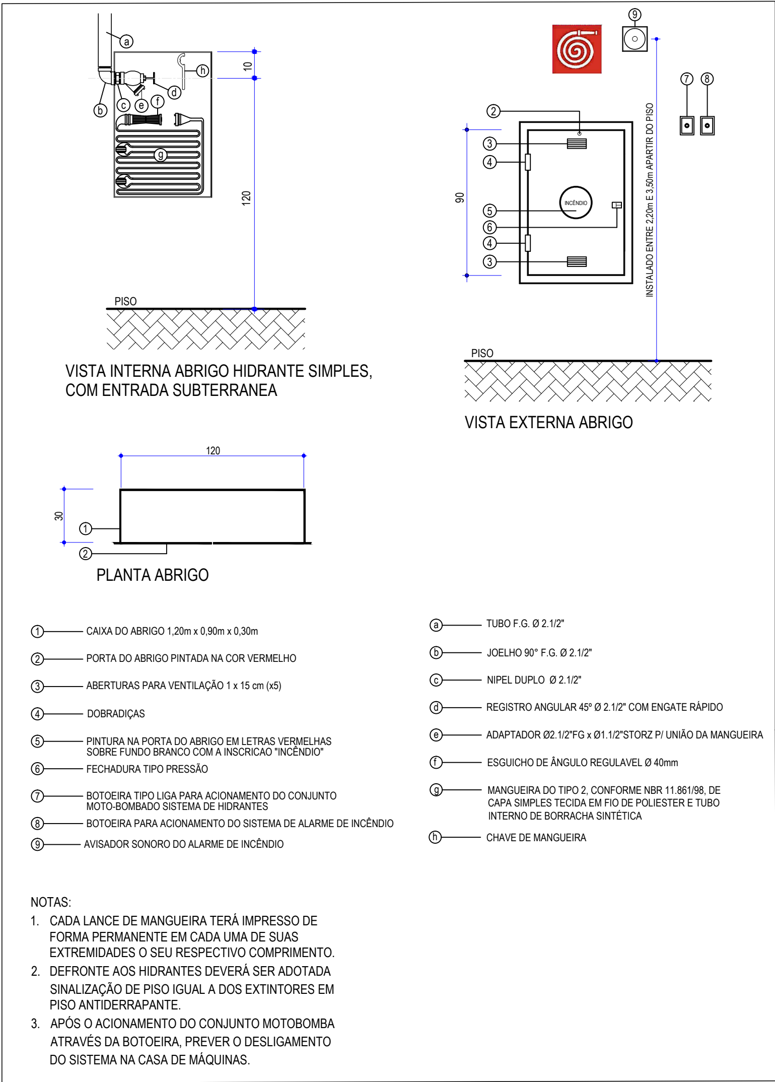
DETALHE DOS HIDRANTES, DA BOTOEIRA DO ALARME DE INCÊNDIO E DO AVISADOR SONORO
