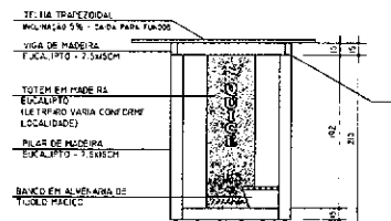
5 ELEVACÃO LATERAL ESCALA 1:50
