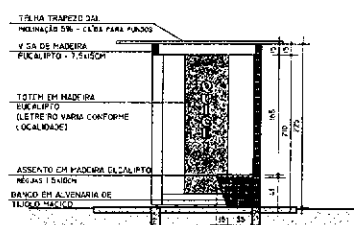
7 CORTES LATERAL ESCALA 1:50
