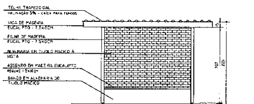
4 ELEVACÃO FRONTAL ESCALA 1:50
