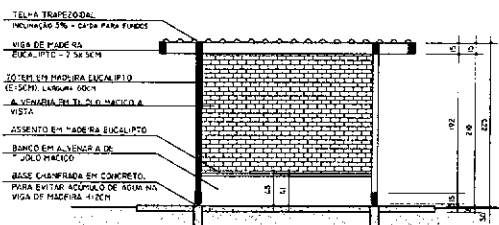
6 CORTES FRONTAL ESCALA 1:50
