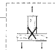
DETALHE DO TIPO DE FIXAÇÃO DAS LIGAÇÕES. UTILIZAR PREGO BITOLA 26x72 7,6x119mm
