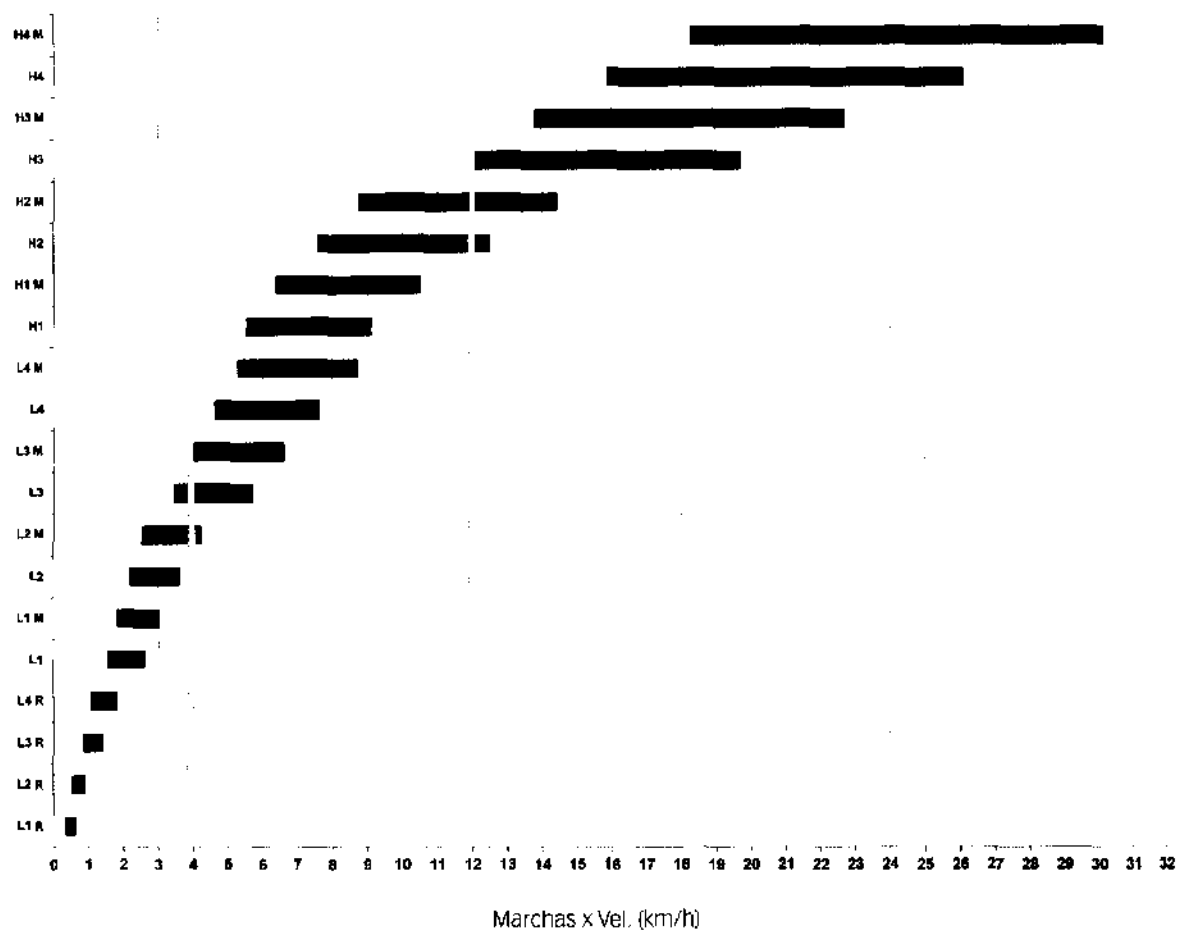
Escalonamento Caixa de Câmbio (Std / Redutor / Multiplicador)
