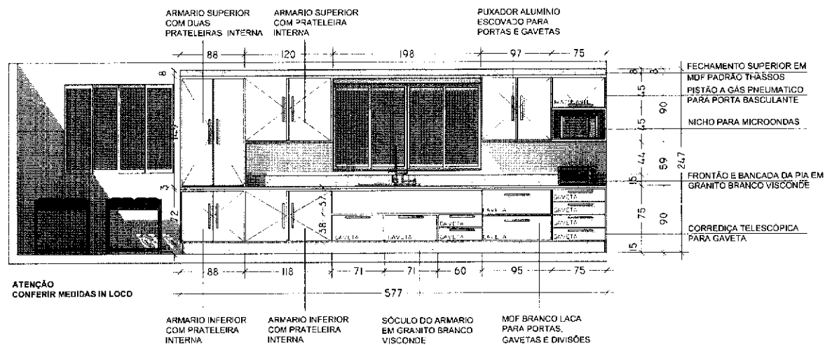
ELEVAÇÃO FRONTAL - PARTE 1 - ESCALA 1:50
