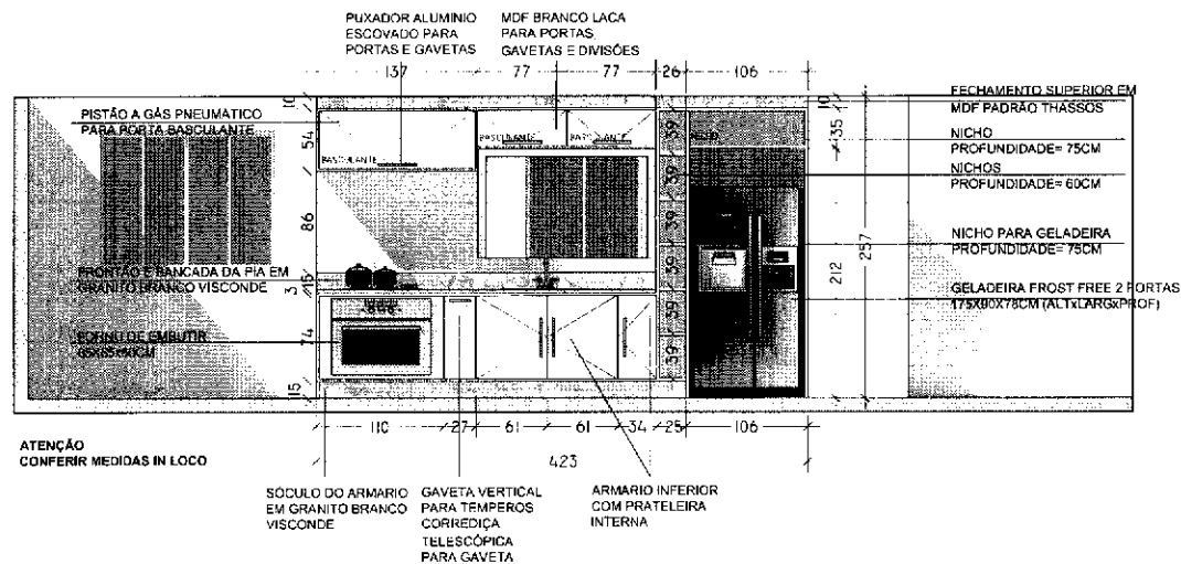
ELEVAÇÃO FRONTAL - PARTE 2 - ESCALA 1:50
