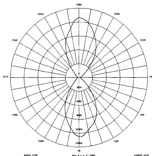
Figura 8 - Curva de intensidade máxima para cada ângulo C (55394-3).
