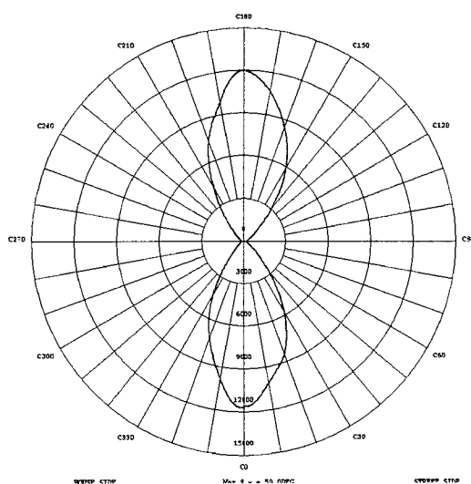
Figura 2 - Curva de intensidade máxima para cada ângulo C (55394-1).
