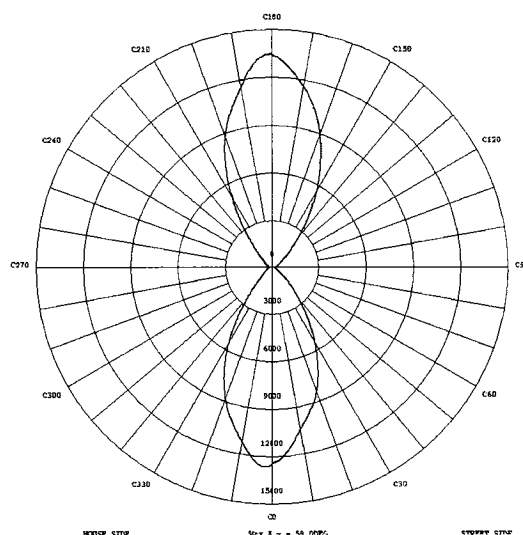
Figura 5 - Curva de intensidade máxima para cada ângulo C (55394-2).
