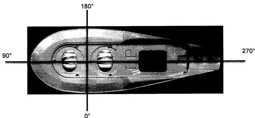
Foto 4 - Eixos Fotométricos
