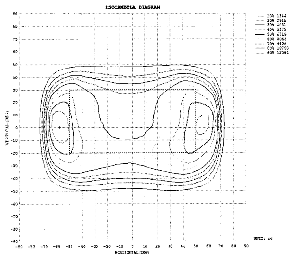
Figura 6 - Curva de distribuição de intensidade (isocandela) (55394-2).
