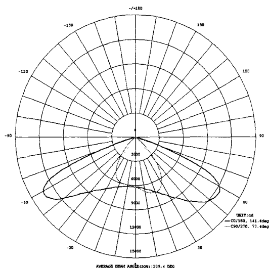
Figura 4 - Curva de distribuição de intensidade luminosa (55394-2).
