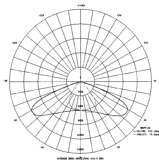
Figura 1 - Curva de distribuição de intensidade luminosa (55394-1).
