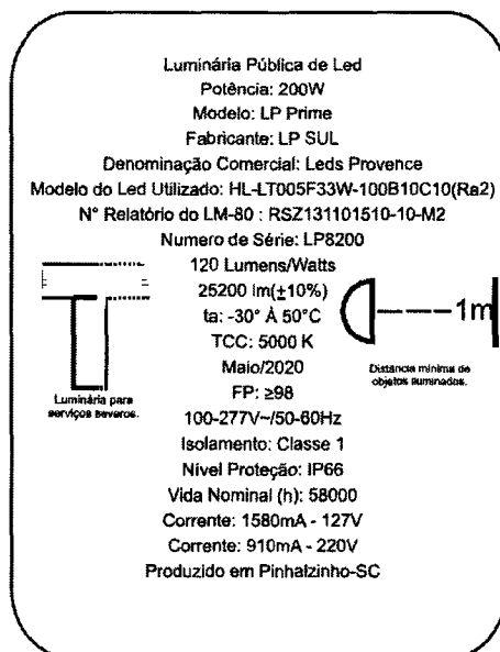
Foto 3 - Placa de identificação da amostra. (Encaminhada via e-mail)
