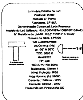
Foto 3 - Placa de identificação da amostra. (Encaminhada via e-mail)
