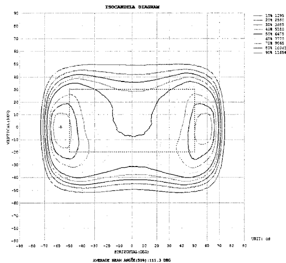
Figura 9 - Curva de distribuição de intensidade (isocandela) (55394-3).
