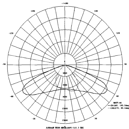
Figura 7 - Curva de distribuição de intensidade luminosa (55394-3).
