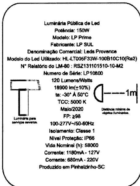
Foto 3 - Placa de identificação da amostra.
