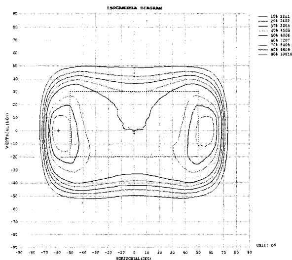
Figura 3 - Curva de distribuição de intensidade (isocandela) (55394-1).
