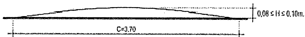
CORTE A-A
