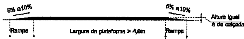
CORTE A-A
