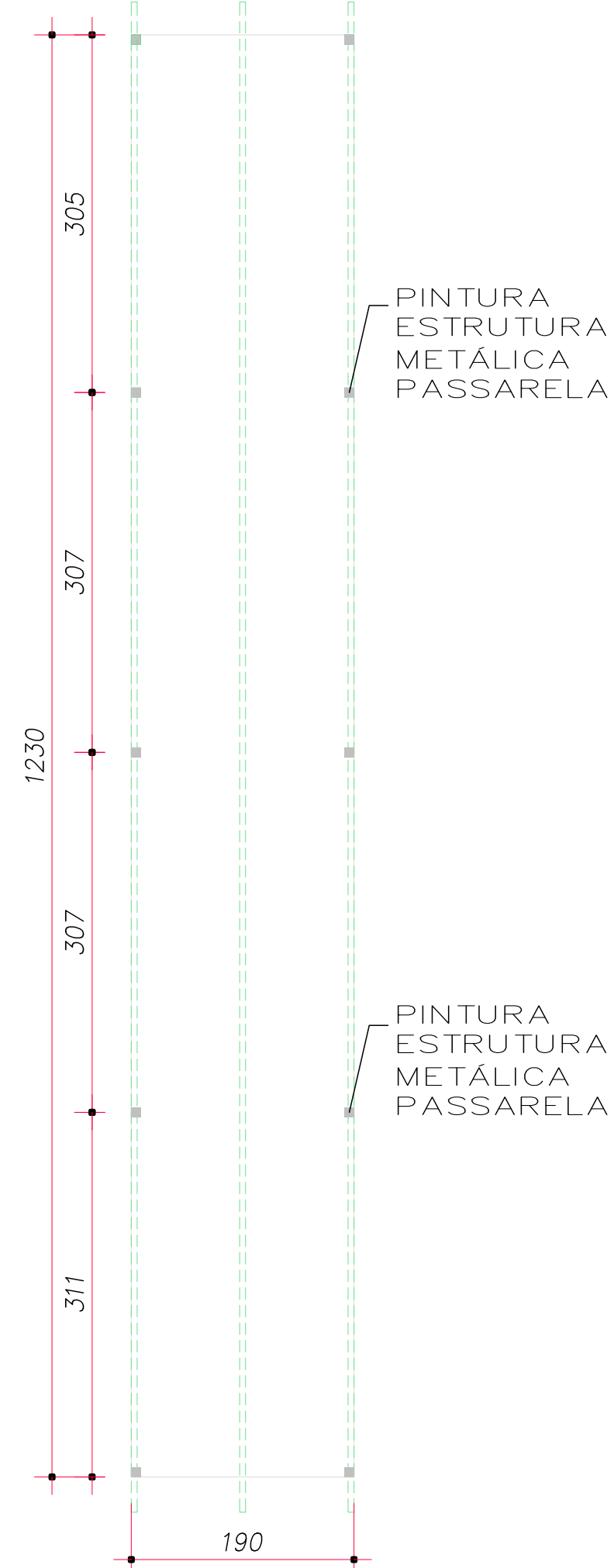
PINTURA PASSARELA COBERTA Escala 1/50
