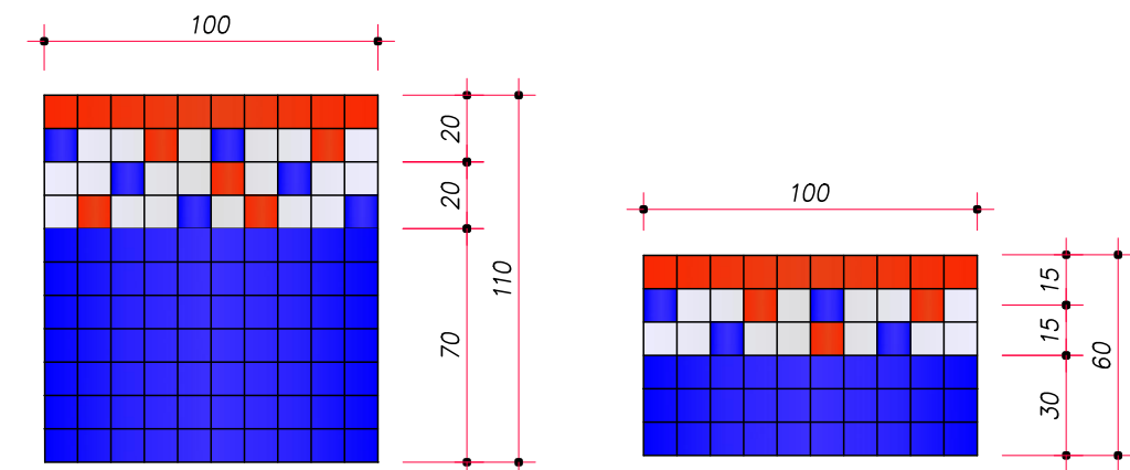
DETALHE PASTILHAS INT/EXT. Escala 1/25
