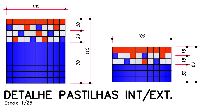
DETALHE PASTILHAS INT/EXT. Escala 1/20
