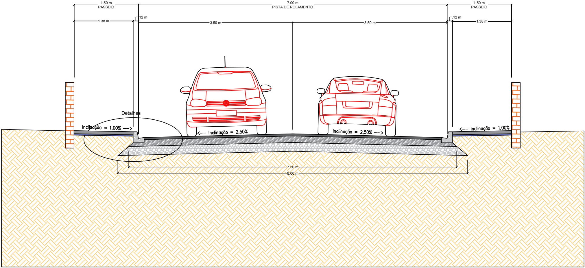
Seção Tipo de Pavimentação Pista 7 m Esc: 1/50
