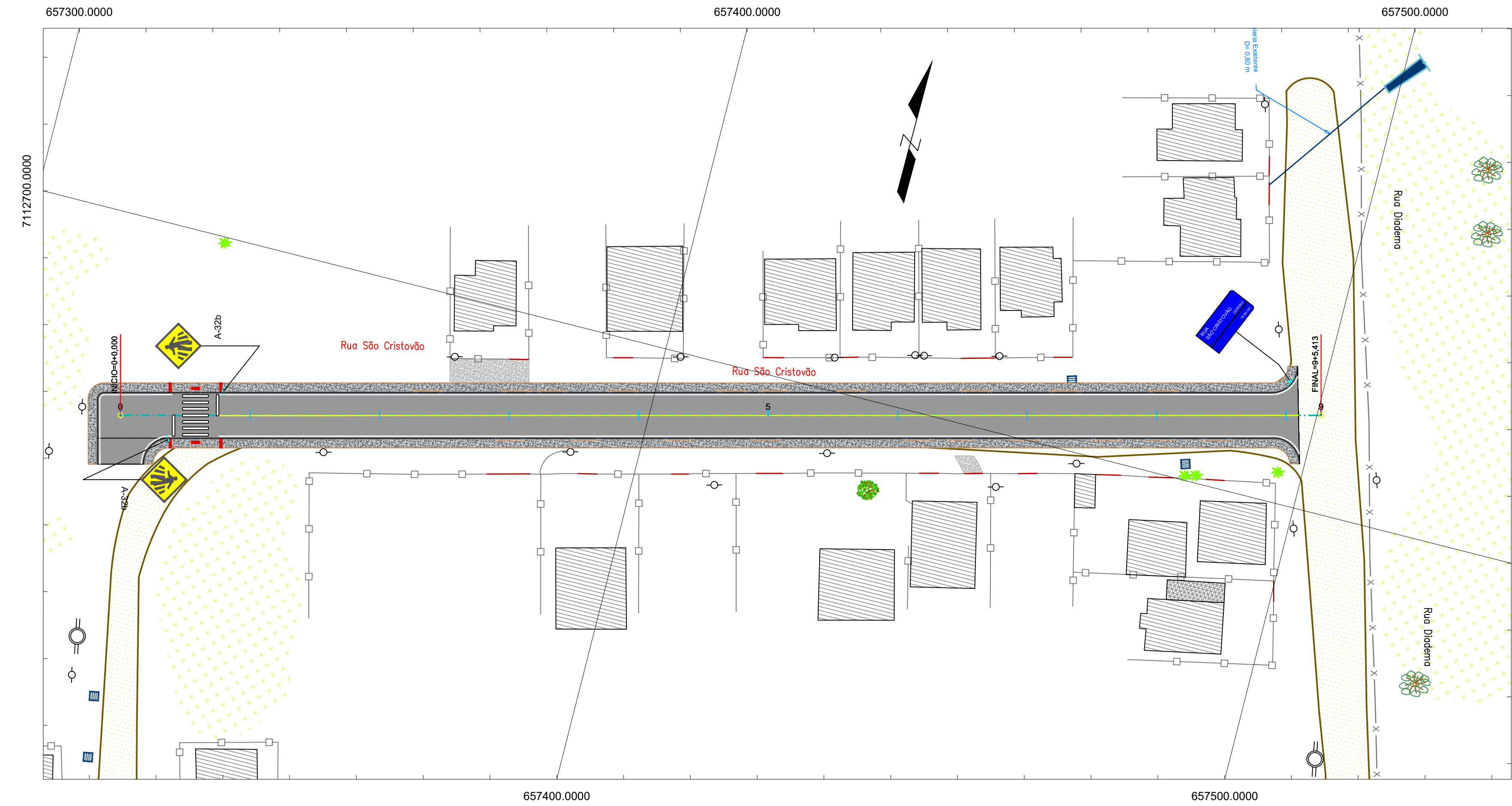
Detalhe Sinalização Horizontal - Pista 7,00 m Faixa de Travessia de Pedestres Tipo Zebrada (FTP-1) Esc = 1:150
