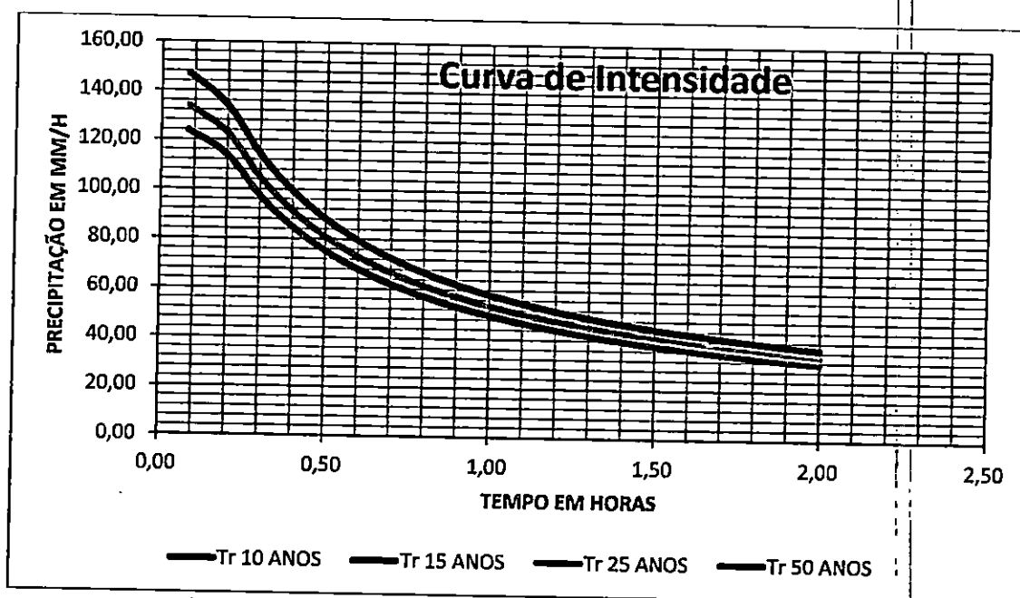
Figura 3-6 – Gráfico de Intensidade da Precipitação
